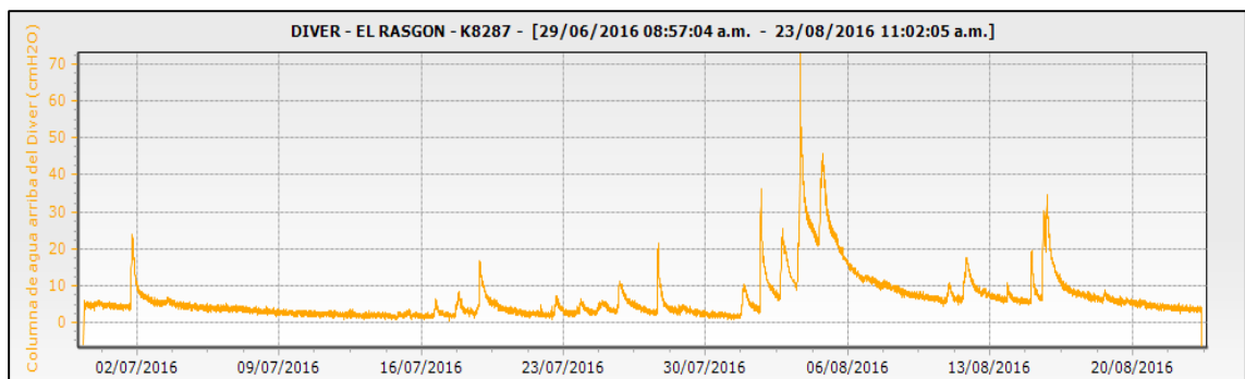
Gráfico 43. Variación columna de agua 29/06/2016 hasta 23/08/2016
