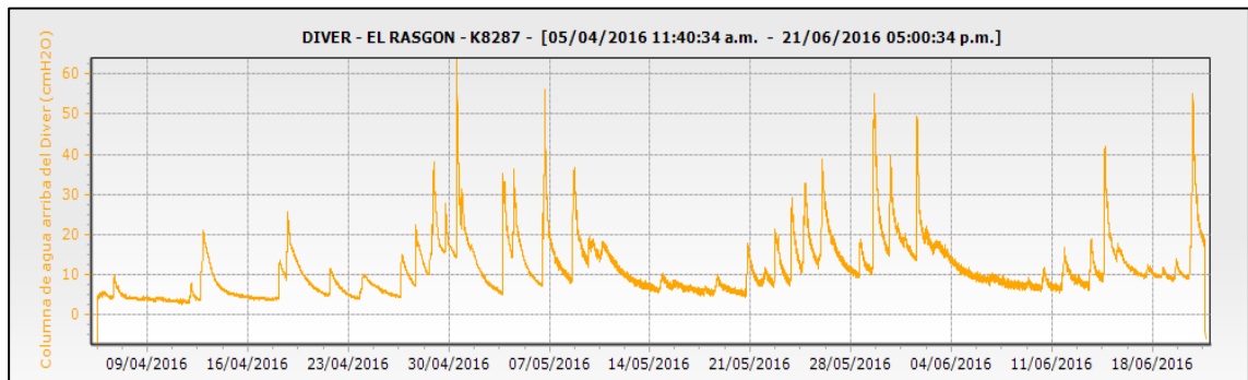
Gráfico 41. Variación columna de agua 05/04/2016 hasta 21/06/2016
